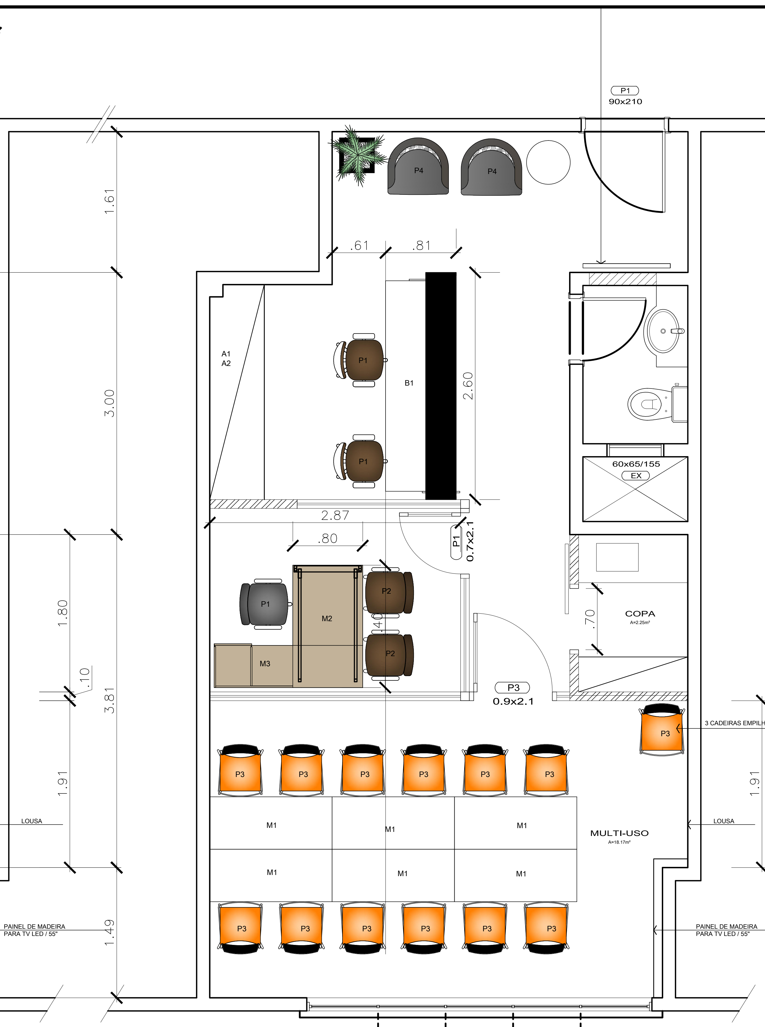
5 PLANTA OPÇÃO 2/LAY-OUT SALA MULTI-USO ESCALA 1 : 25
