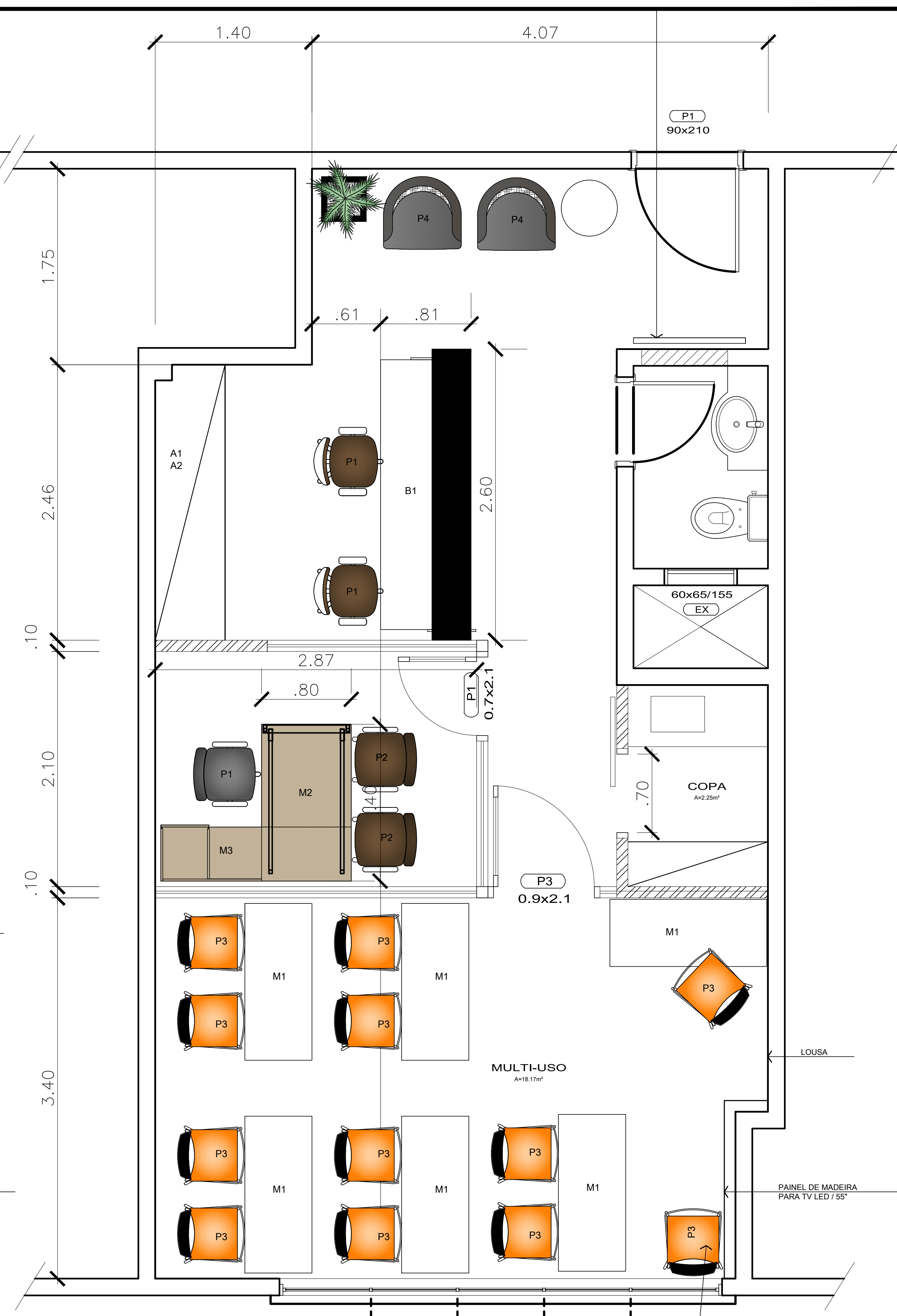
5 PLANTA OPÇÃO 3/LAY-OUT SALA MULTI-USO ESCALA 1 : 25
